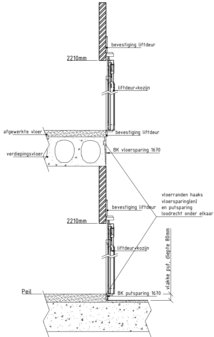
Doorsnede principe aansluiting A-deur in bouwkundige sparring
