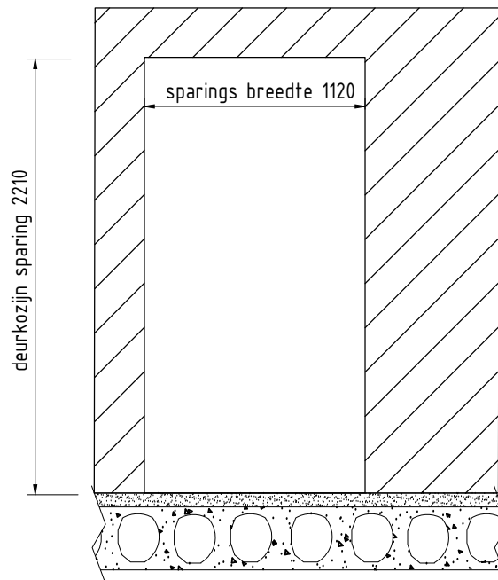
Deursparingen in de wand
