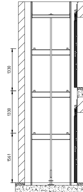
aanzicht B
