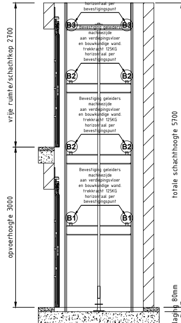
aanzicht D
