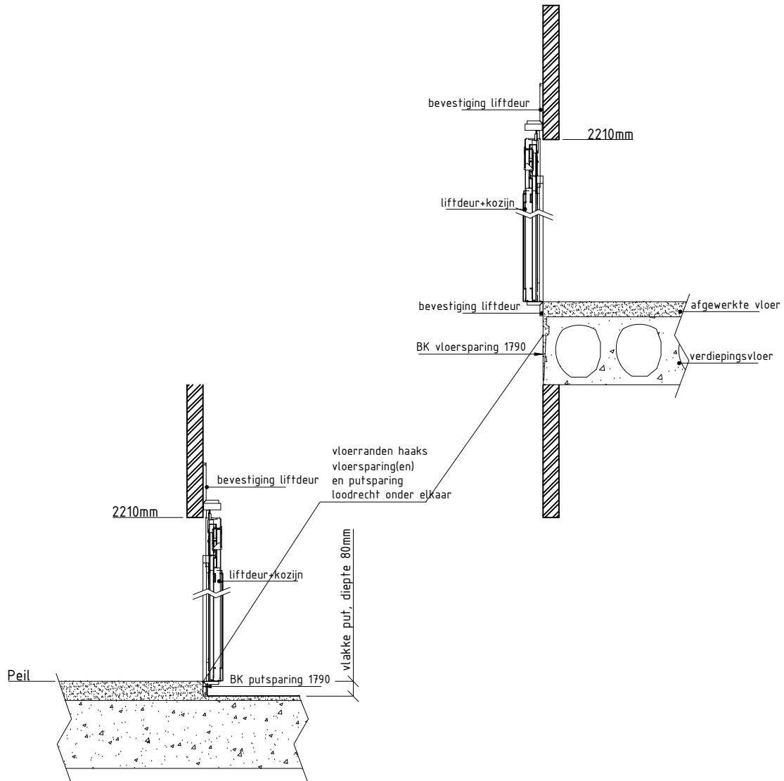
Doorsnede principe aansluiting A-deur in bouwkundige sparring
