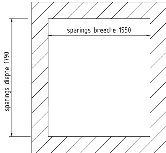
Sparing(en) in de vloer(en)
