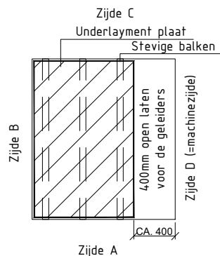
Door derden aan te brengen: Tijdelijke werkvloer ter hoogte van de verdiepingsvloer(en)
