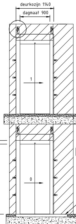
aanzicht A
