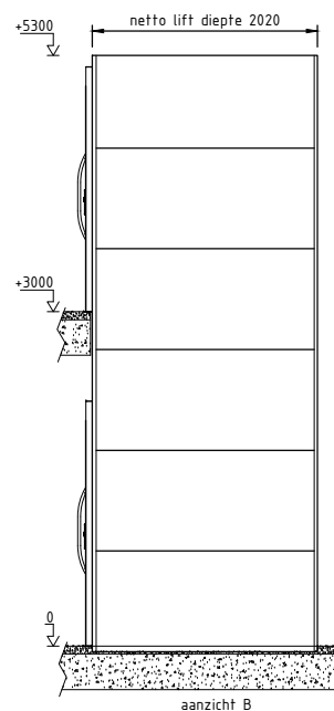
aanzicht B
