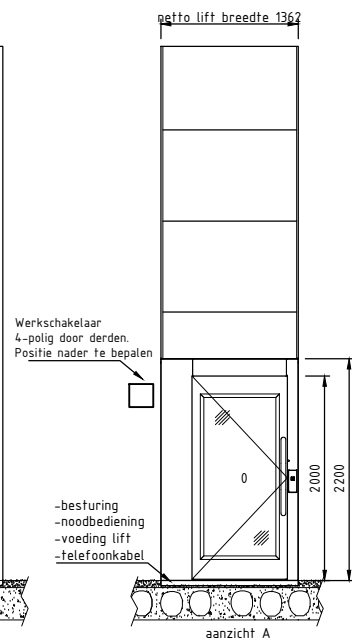
aanzicht A
