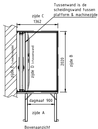
Bovenaanzicht
