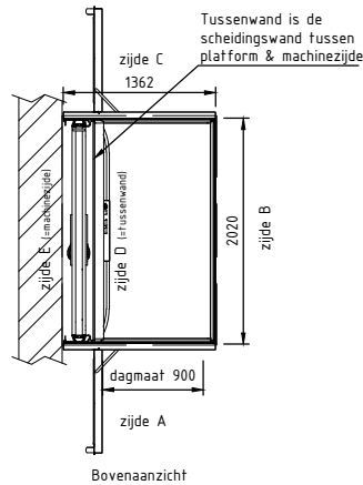
Bovenaanzicht
