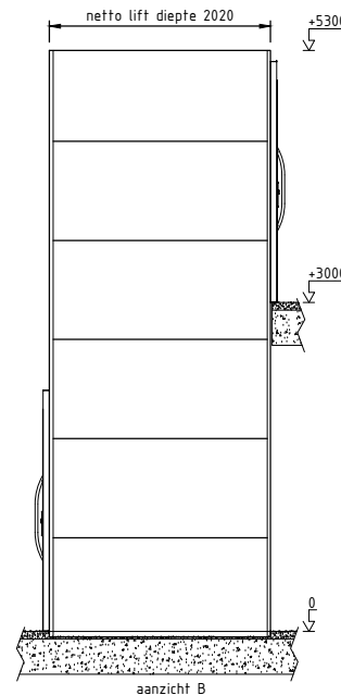
aanzicht B
