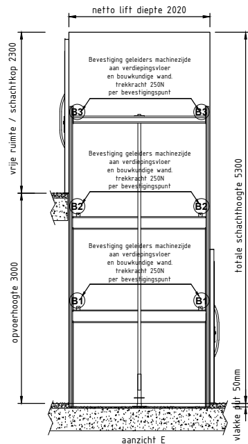
aanzicht E
