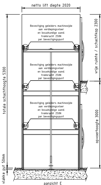
aanzicht E
